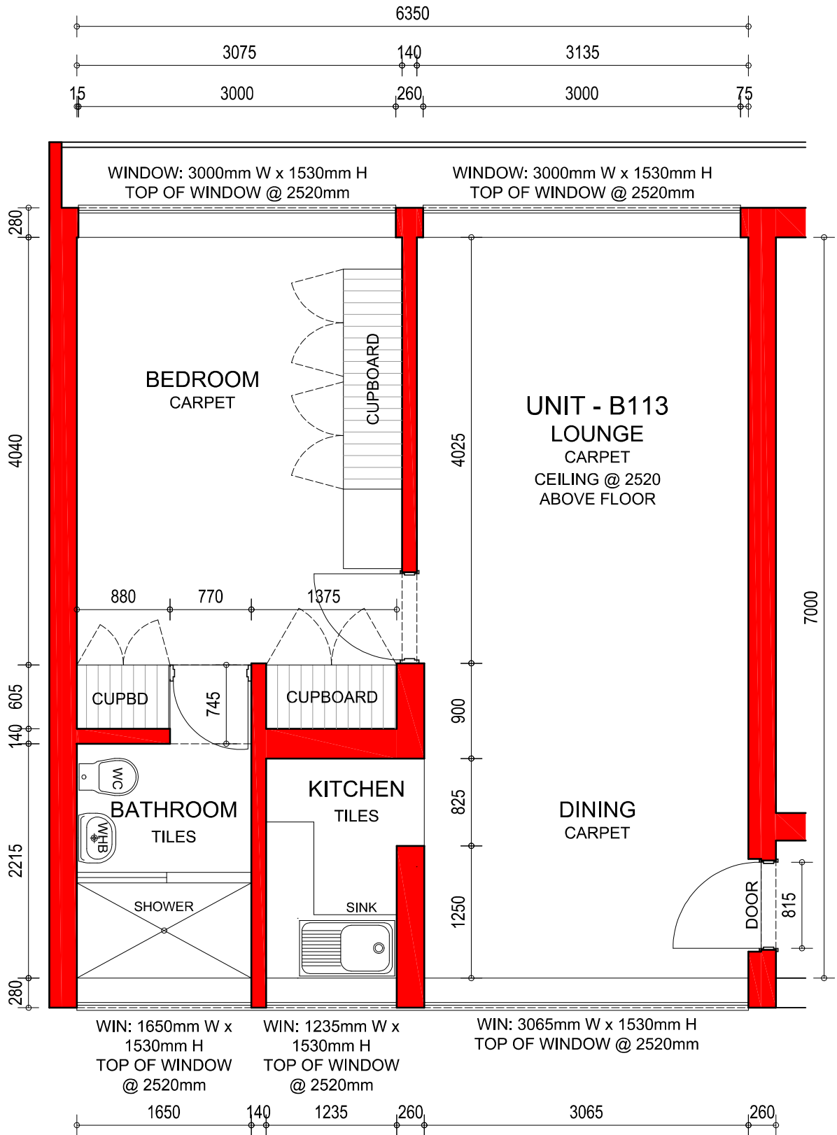
UNIT B113 : PLAN SCALE 1:50
