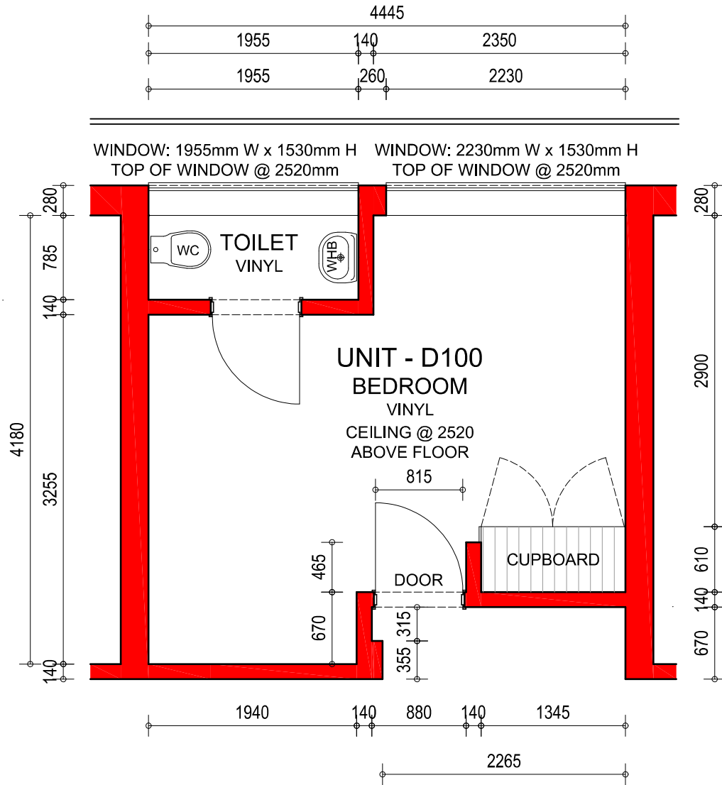
UNIT D100 : PLAN SCALE 1:50
