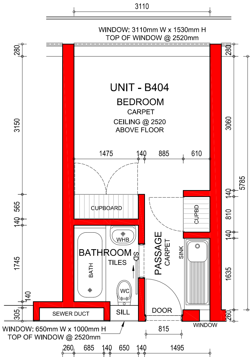
UNIT B404 : PLAN SCALE 1:50
