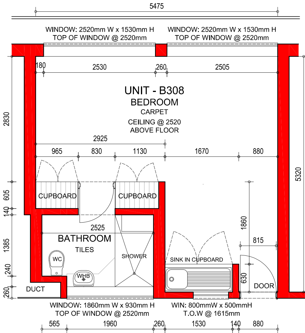
UNIT B308 : PLAN SCALE 1:50
